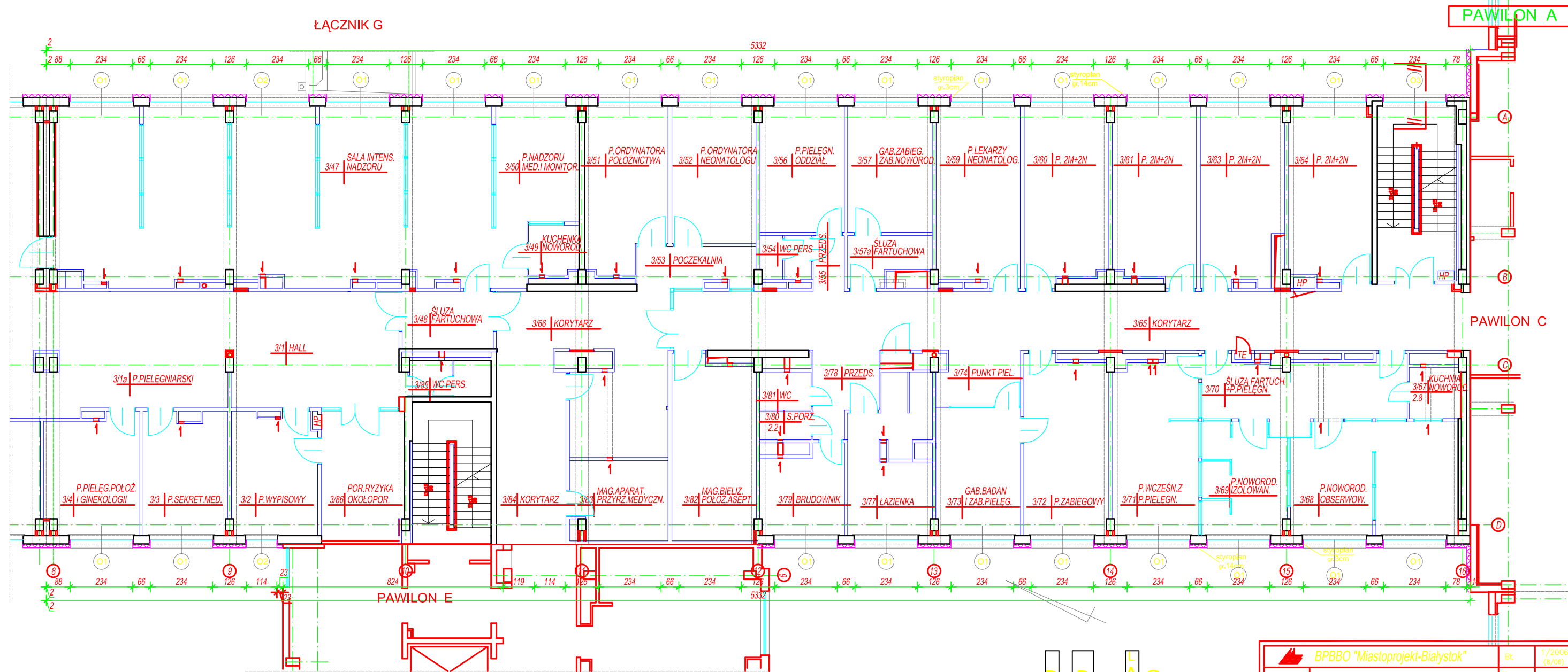
RZUT PIĘTRA II STRONA PRAWA skala 1:100 BUDYNEK GŁÓWNY - PAWILON A
